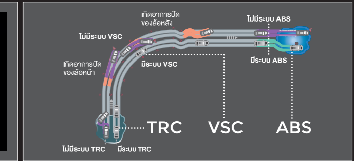
TRC (Traction Control System) ระบบป้องกันล้อหมุนฟรี VSC (Vehicle Stability Control) ระบบควบคุมการทรงตัว ABS (Anti-lock Brake System) ระบบป้องกันล้อล็อก EBD (Electronic Brake-force Distribution) ระบบกระจายแรงเบรก BA (Brake Assist) ระบบเสริมแรงเบรก
