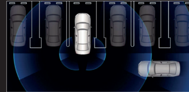
REAR CROSS TRAFFIC ALERT ระบบช่วยเตือนชน-ถอยรถ
